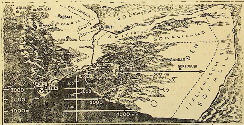
Relieful părții de NE a Abisiniei. Ce e alb sunt locurile joase; cu cât liniile sunt mai desc, cu atât locul e mai înalt. Partea neagră arată secțiunea în mijlocul pământului abisinian cu groapa în care e linia ferată.
