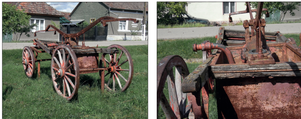
Fig. 484 a - b. Șoșdea (jud. Caraș-Severin). Pompă manuală montată pe trasură hipo expusă în preajma Primăriei într-o stare de conservare lamentabilă (Foto: 2014)
