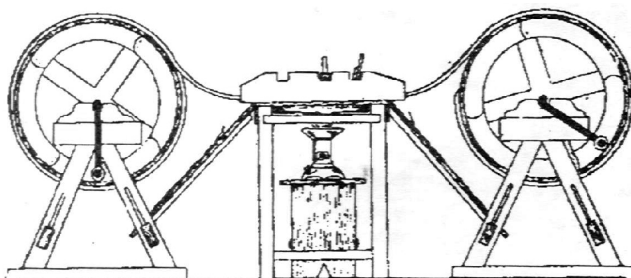
Instalație pentru confecționarea lumânărilor prin îmbăiere
