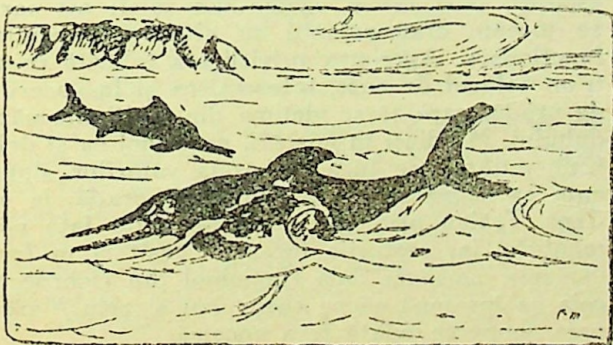
Fig. 4. Ichthyosaurus.
