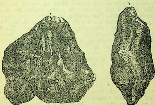
Fig. 2.—Un meteorit văzut din față și dintr'o coastă.
