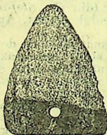
Fig. 1. — Un vârf de lance făcut dintr'un meteorit.
