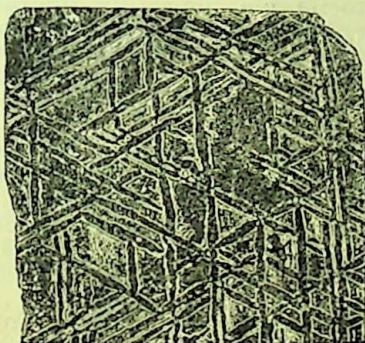
Fig. 6. — Figurile văzute într'un fer meteoric luciat.
