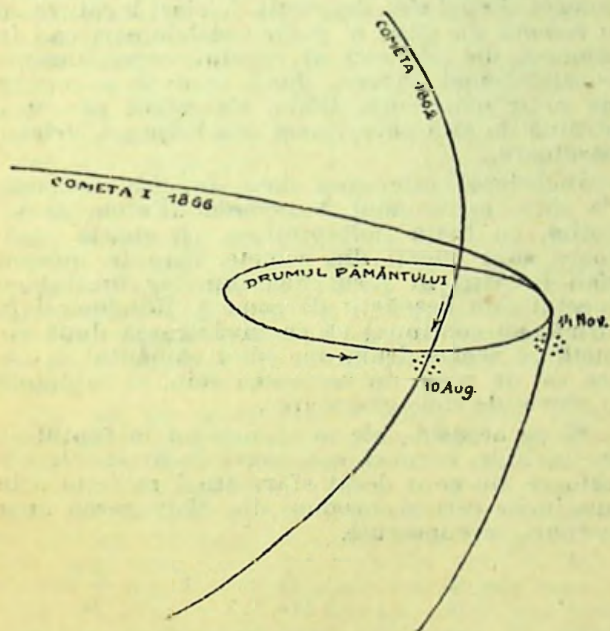
Fig. 7. — Incrucișarea drumurilor a 2 comete cu drumul pământului în jurul soarelui, tocmai în locurile unde se văd pe cer nouri de stele căzătoare.
