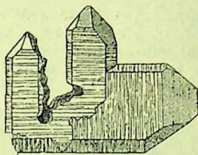
Fig. 3. — Cristali de cuarț.
