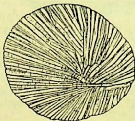
Fig. 5.—Structura fibroasă a unci broboane din meteorit.
