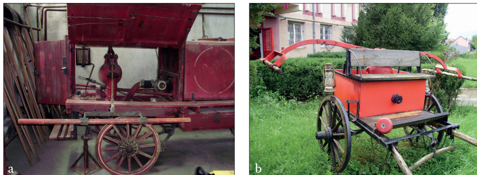
Fig. 541 a - b. Lugoj (jud. Timiș) . Atelaje vechi păstrate ca „piese de muzeu” la Detașamentul de Pompieri, a) Pompă tip „Timișoara” adusă de la Balinț; b) Pompă manuală cu balansier rabatabil, tip „Aiud” (Foto: Dorina Rusu, 2014)
