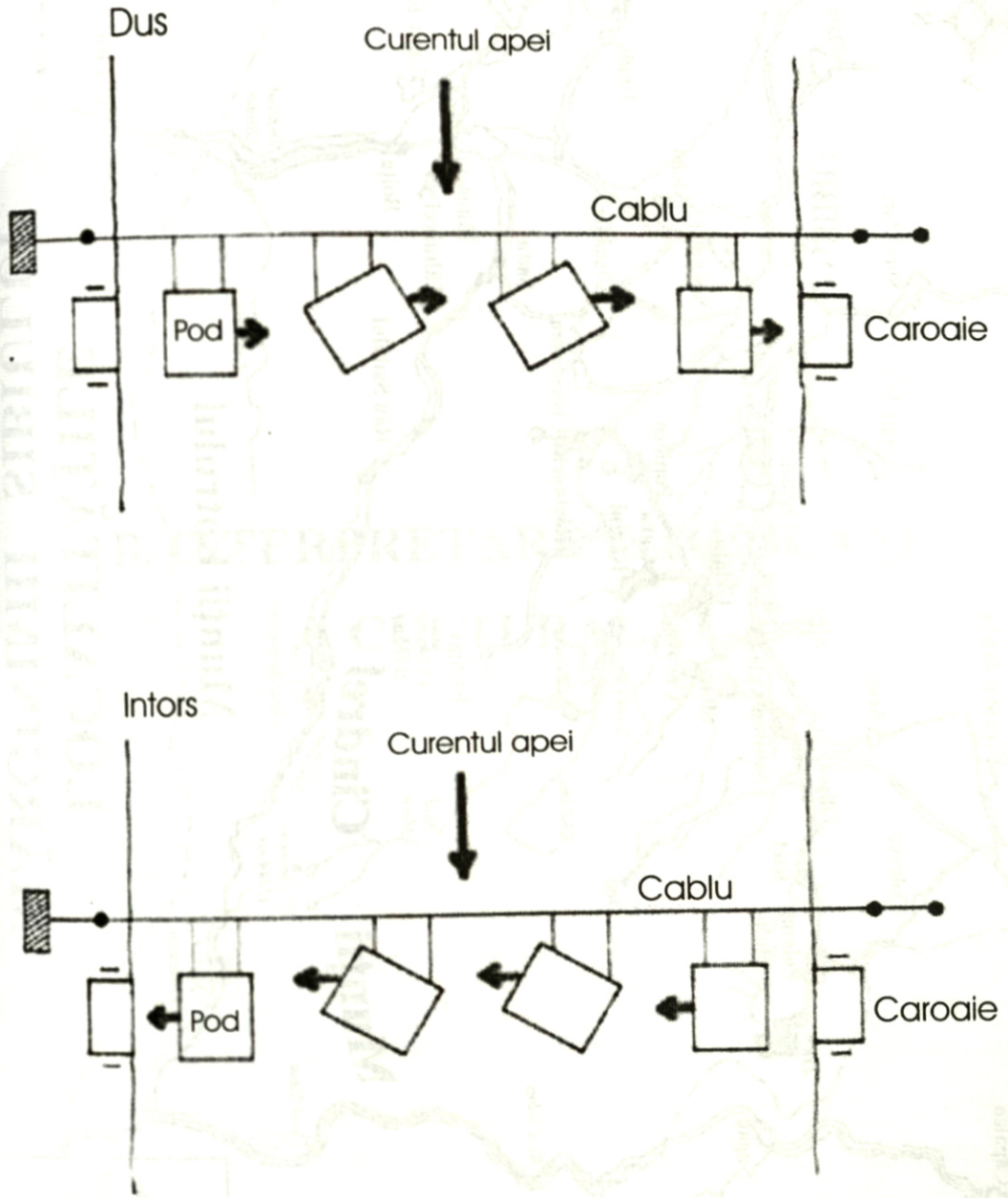
Pod plutitor pe cablu (de pe Olt) - Turnu Rosu - Schema de functionare-
